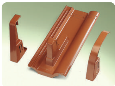
ОПОРНА ЧЕРЕПИЦЯ ПІД КОЛОДУ АБО СНІГОЗАТРИМУЮЧУ РЕШІТКУ
